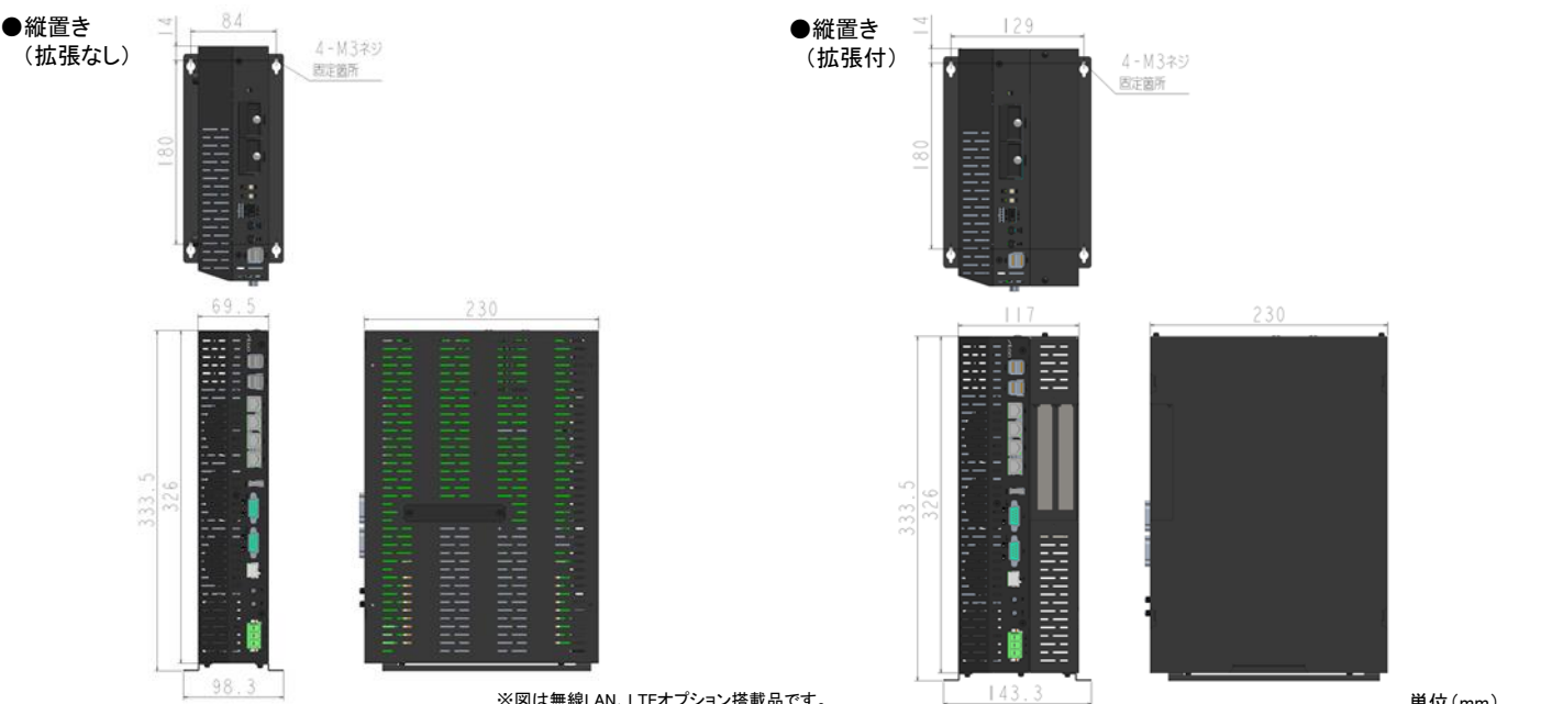
※図は無線LAN、LTEオプション搭載品です。 ファン搭載モデルとファン非搭載モデルでは筐体のスリット数が異なります。
